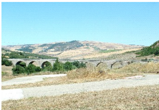
Il ponte a dieci luci della SS 90 bis, che scavalca, a Santo Spirito, il torrente della Ginestra, dove morirono, per incidente sul lavoro, nel 1950, Antonio Chiuchiolo e Gaetano De Florio.
